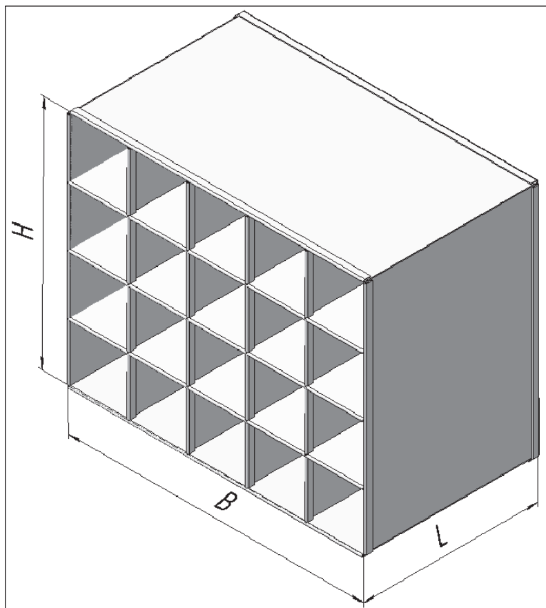
Рисунок 2 - Проходка типа ПК-4/5-0,4x0,5x0,3
